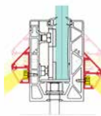
LED sur l'extérieur et l'intérieur
