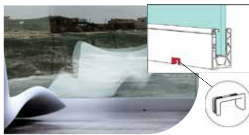
Profilé avec fraisage traversant
