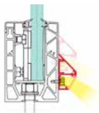
LED sur l'extérieur
