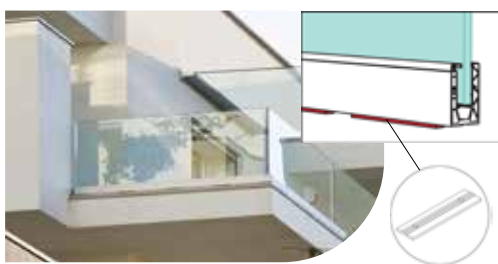
Cales en aluminium
